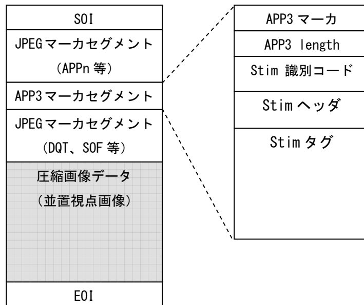
図 2 Stim タグを含む本体画像ファイルの構造
